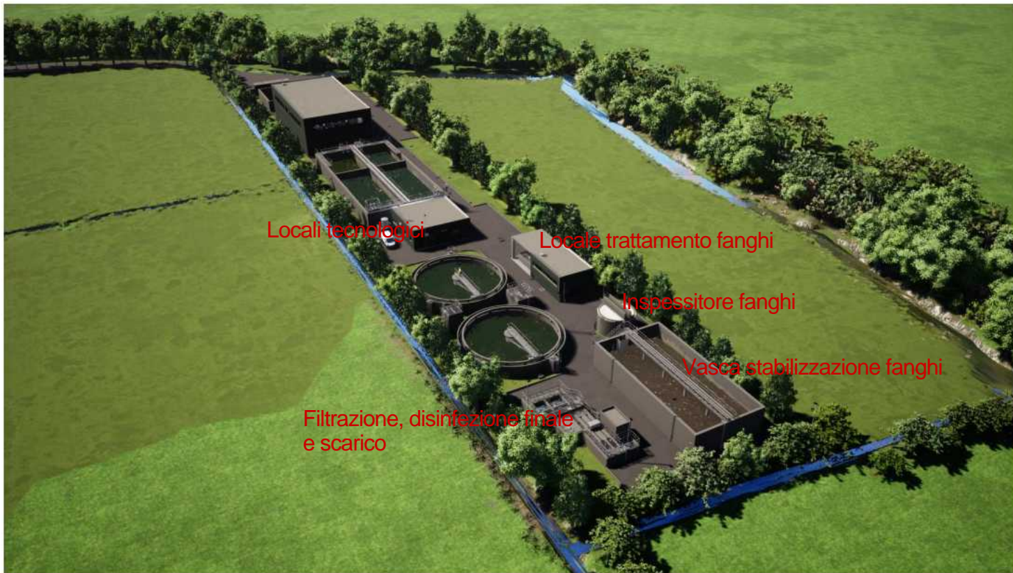
Nuovo depuratore di Calvisano (BS) Vista Sud-Ovest
